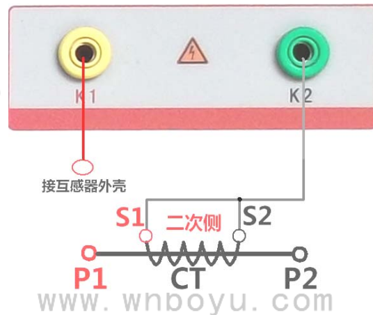
图 19, CT 交流耐压接线图
