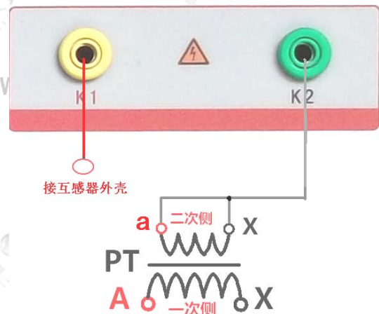
图 33，PT 交流耐压接线图
