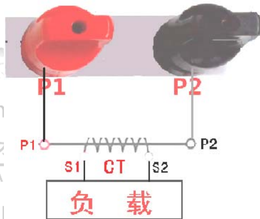
图 17、CT 一次通流接线图
